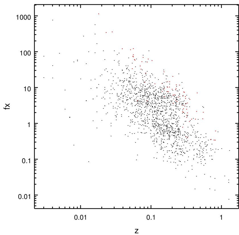
bax.lis
